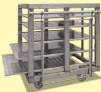
Carrello di caricamento con lamiere estraibili
